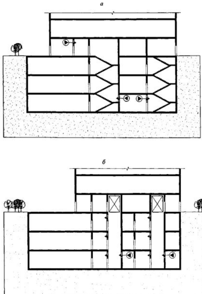
Рис. 5. Схемы подачи воздуха в лестничные клетки (а) и в лифтовые шахты (б) подземной части здания
